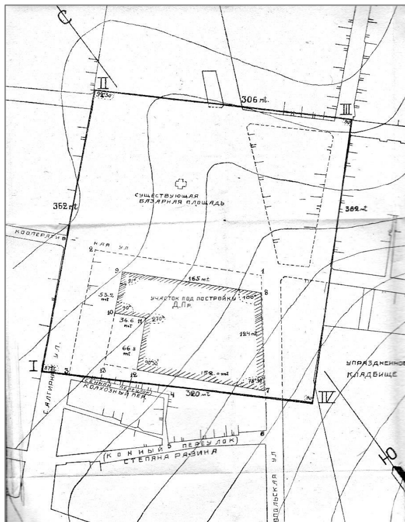
Фрагмент «Плана Правительственной площади и участка под постройку Дома правительства Крымской АССР в г. Симферополе».
