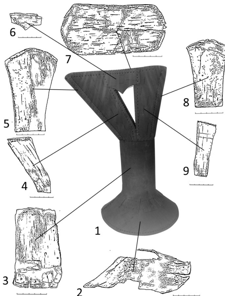
Рис. 1. Реконструкция берестяного каркаса боки из могильника Телеутский Взвоз-1 с подетальным расположением всех частей: 1 – реконструкция каркаса, 2 – воронкообразное расширение, 3 – трубочка (цилиндр, колонна), 4 – боковая передняя наклонная полоса (2 шт.), 5 – лицевая панель, 6 – пятиугольная фигурная пластинка (2 шт.), 7 – крышечка, 8 – тыльная панель, 9 – боковая задняя наклонная полоса (2 шт.).
