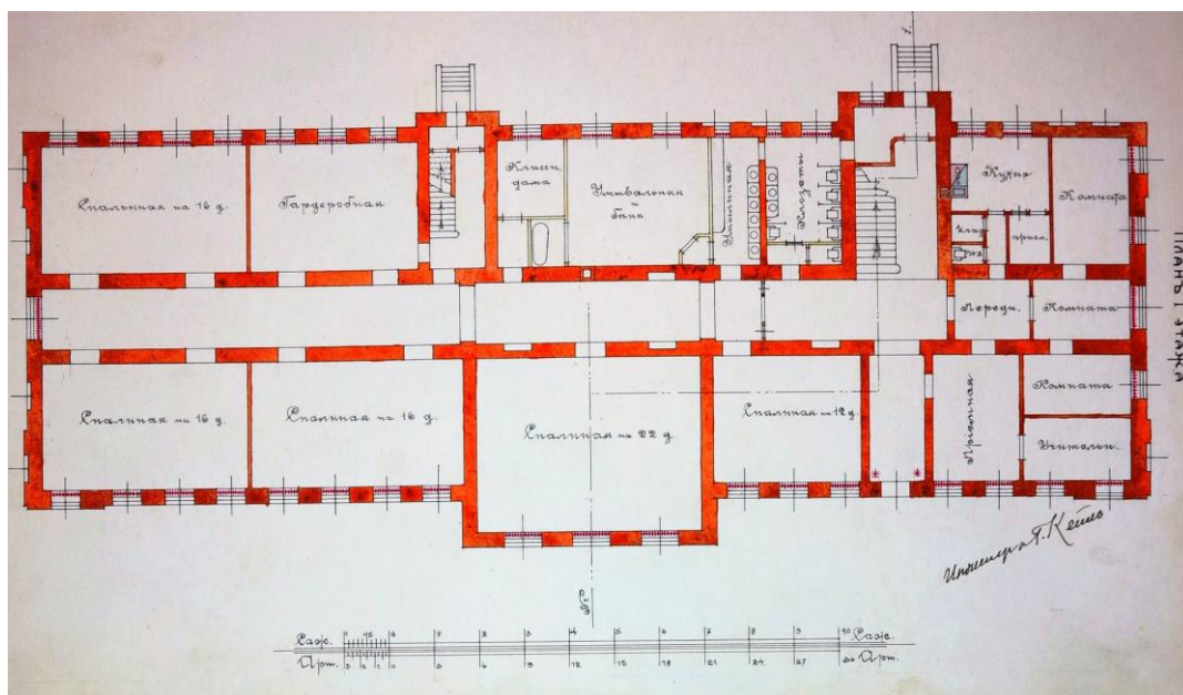
План 1-го этажа Окречского женского высшего начального училища
