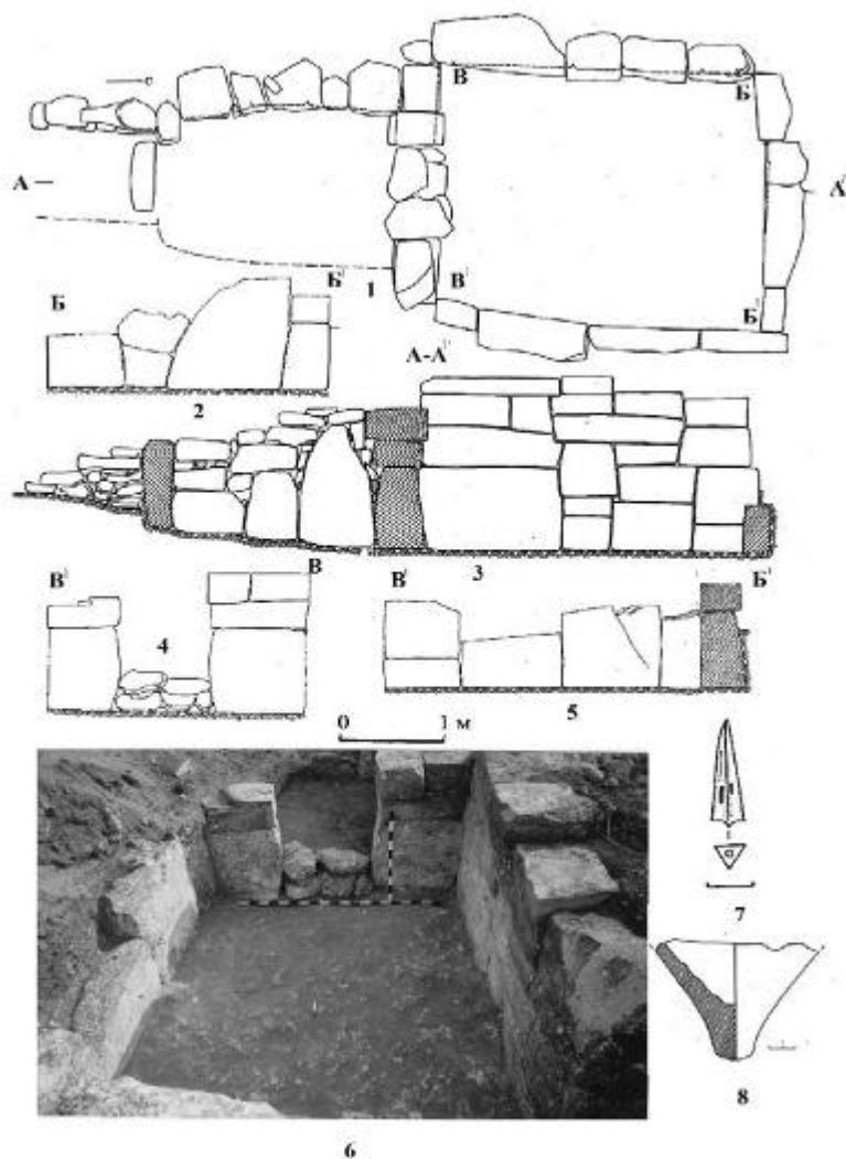
Рис. 5. Курган 2, основное погребение. 1–5 – план и фасировки склепа. 6 – вид из погребальной камеры на входной проем. 7 – наконечник стрелы. 8 – ножка синопской амфоры.
