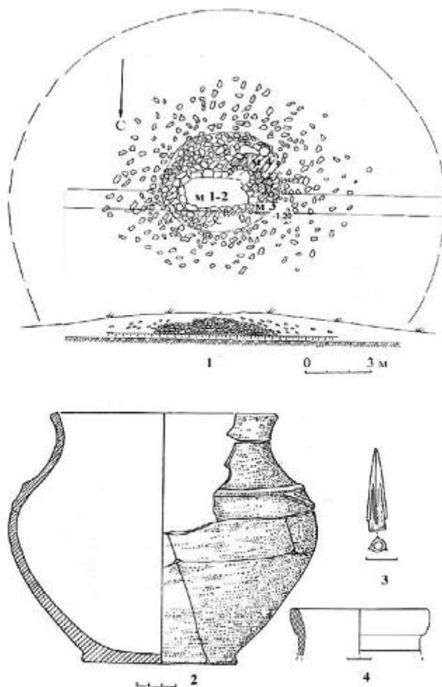
Рис. 4. Курган 1. 1 – план и стратиграфия кургана. 2 – лепной сосуд из погребения 2. 3 – наконечник стрелы из заполнения погребения 1. 4 – венчик амфоры из насыпи кургана.
